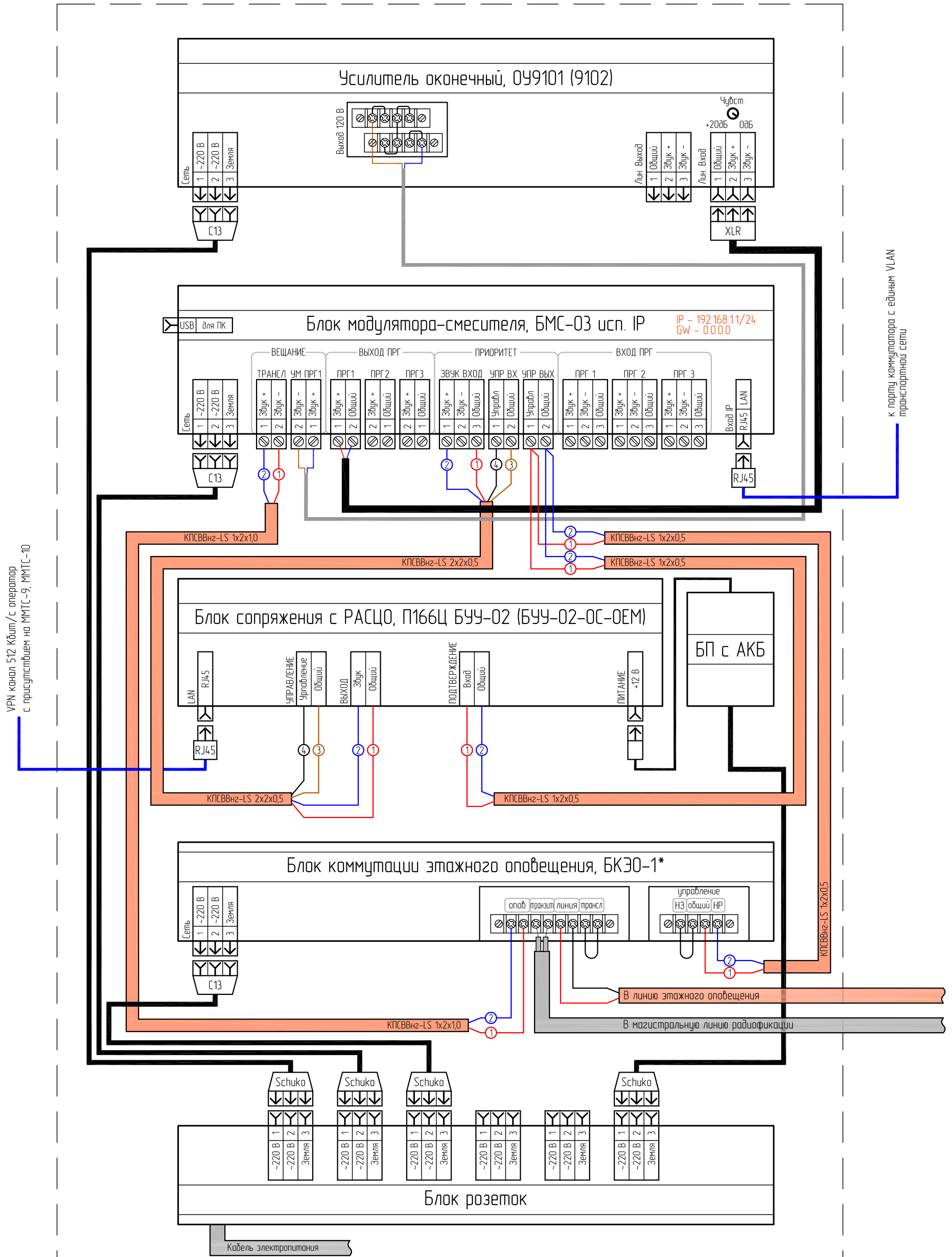
Устройство подачи программ вещания УПВ 1918 М1 исп. IP (ПОСЛЕДУЮЩИЙ)
