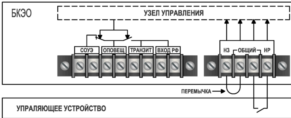
Схема подключения БКЭО с нормально-разомкнутым контактом управления.
