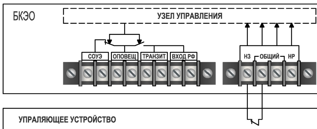
Схема подключения БКЭО с нормально-замкнутым контактом управления
