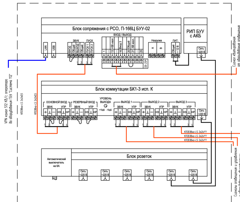
Устройство сопряжения с РСО УС-3 (с БУУ-02) схема соединения блоков
