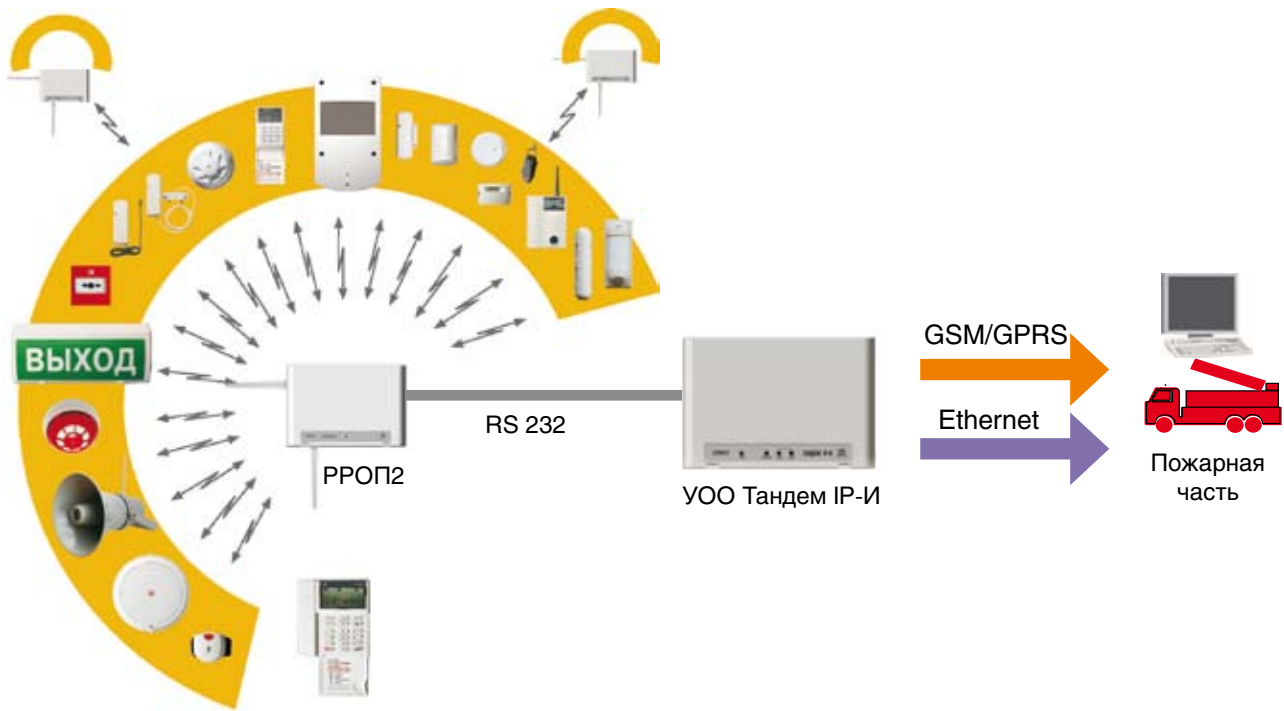
Рис.17. Пример подключения по протоколу RS-232 (ВОПС «Стрелец»)
